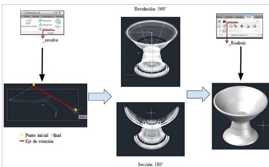
Figura 4. Esquema de pasos para para obtener objetos completos en 3D a partir del comando Revolución hasta llegar ha sombreado esquemático. Fuente: Elaboración Autores
