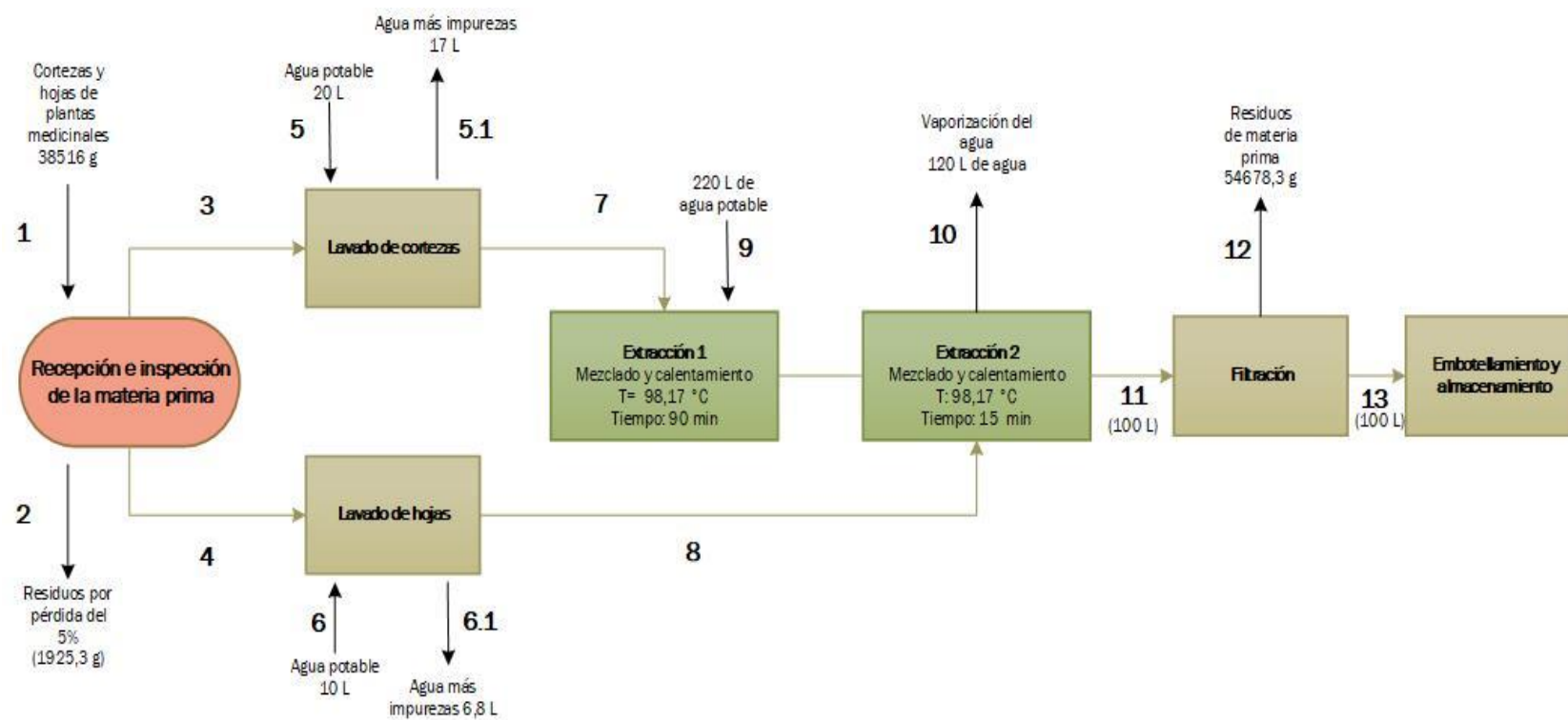
Figura 1. Diagrama de bloques del proceso para la elaboración de jarabe terapéutico diseñado para el cantón Arajuno. Realizado por: Barrionuevo, Jair, 2022
