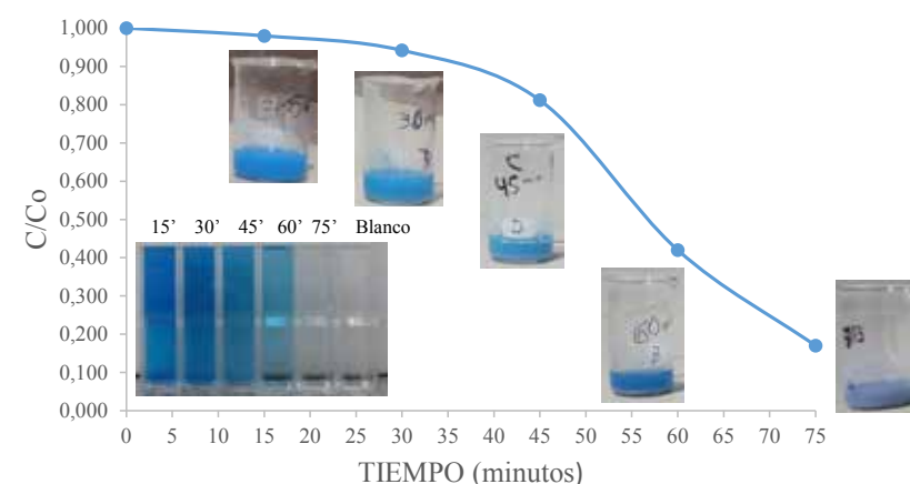
Figura 3. Fotodegradación de azul de metileno con TiO_2 .
