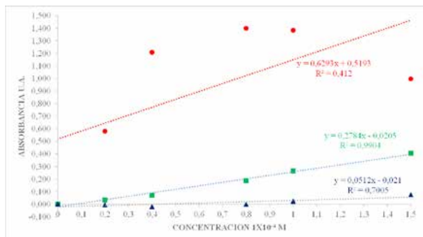
Figura 2. Curvas de calibración de azul de metileno utilizando el análisis de fotografías RGB. Círculos (usando el color rojo) cuadrados (usando el color verde), triángulos (usando el color azul).
